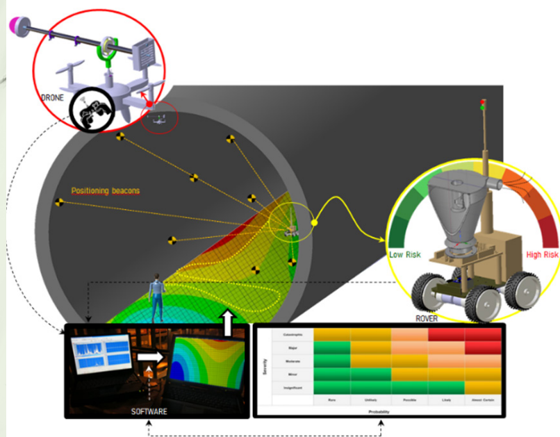
Prototipo digital del funcionamiento de la nueva plataforma PRACAN.
